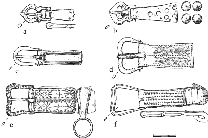
4. attēls. Jostas sprādzes ar sprādžu gala apkalumiem (zīm. Aiga Ivbuļe).
